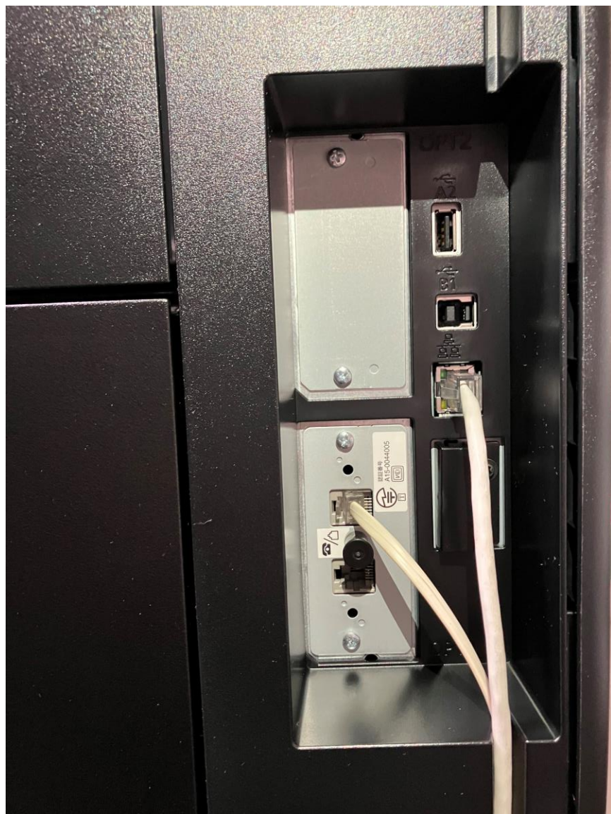
【LAN・FAXケーブル接続】
